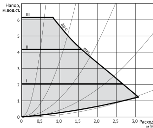
Гидравлические характеристики циркуляционного насоса Wilo Para 25-130/6-43/SC-12#WRU
